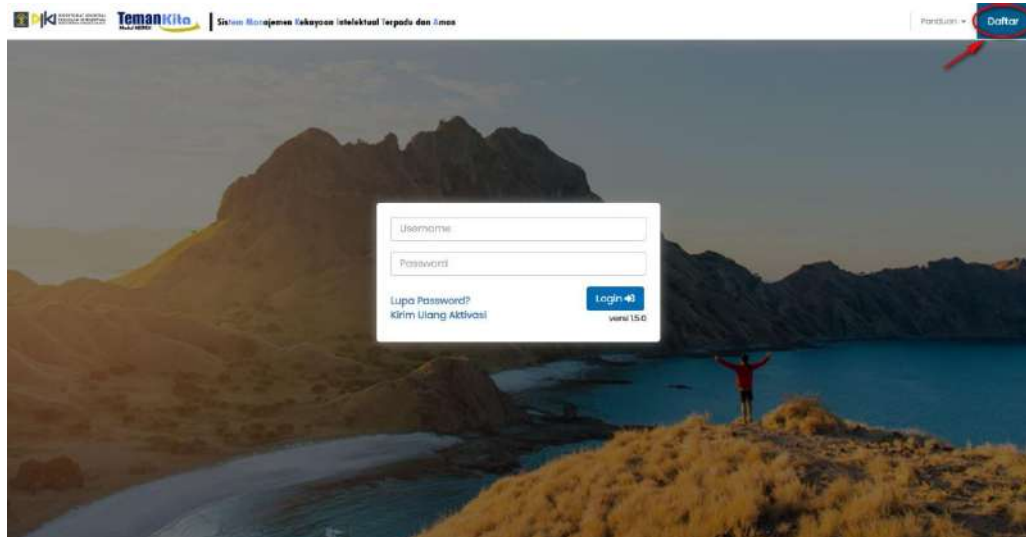
Gambar 1 Halaman Login
