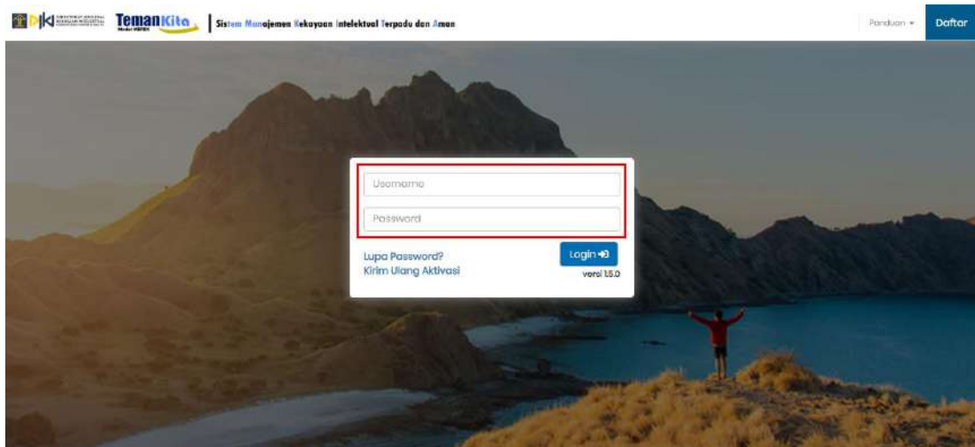
Gambar 11 Halaman Login
