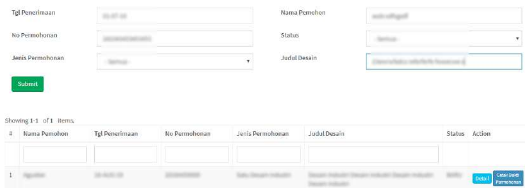
Gambar 40 Pencarian Permohonan
